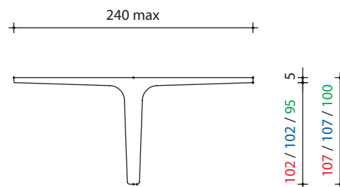
SEZIONE A-A
