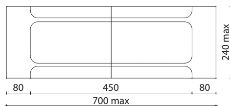
PIANTA CAPRIATA "DI TESTA"
